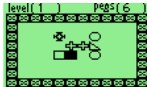
Figure 12.12.: pegbox
