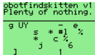
Figure 10.15.: Robotfindskitten
